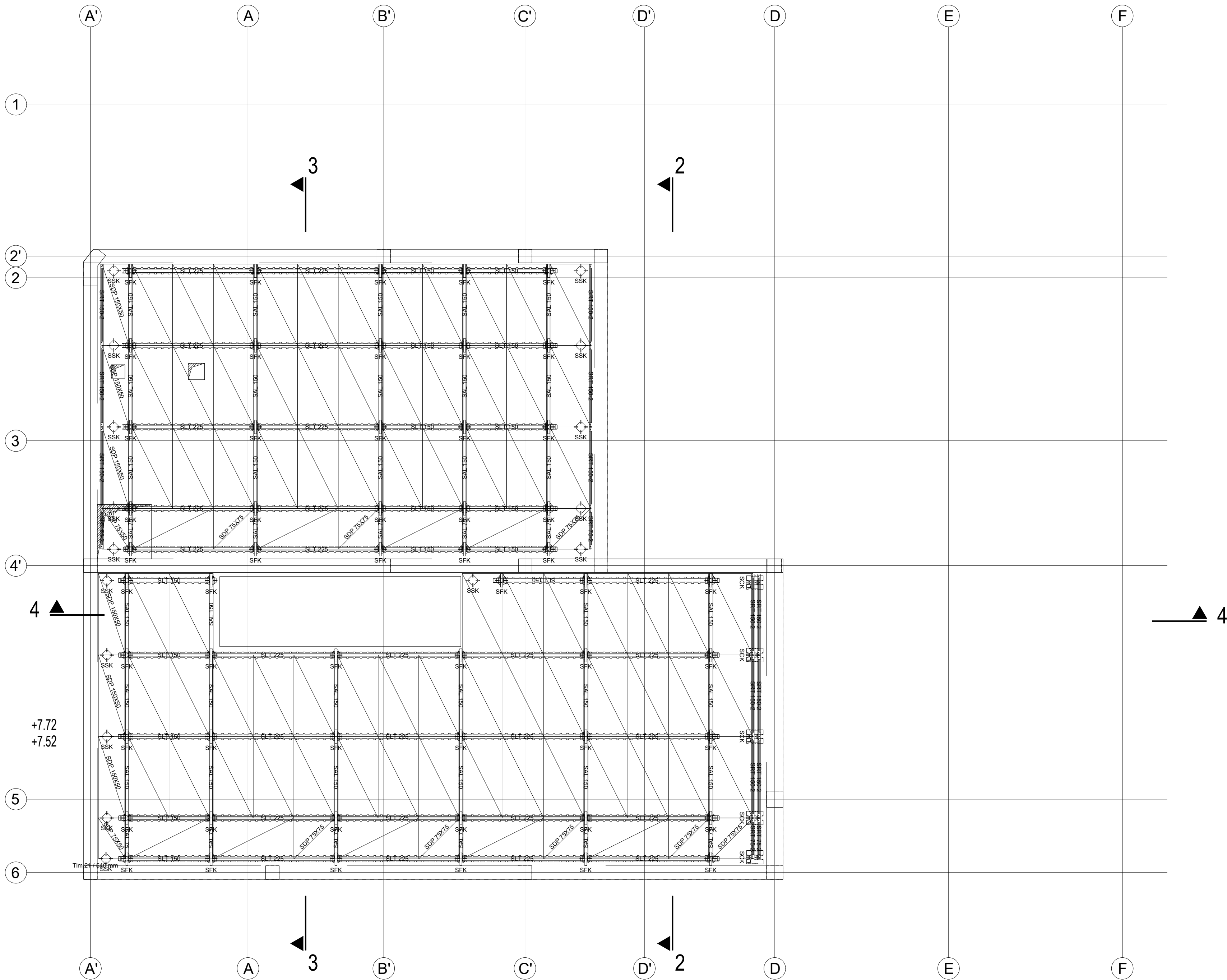
PLAN OPLATE PLOČE POS 201 1:50
