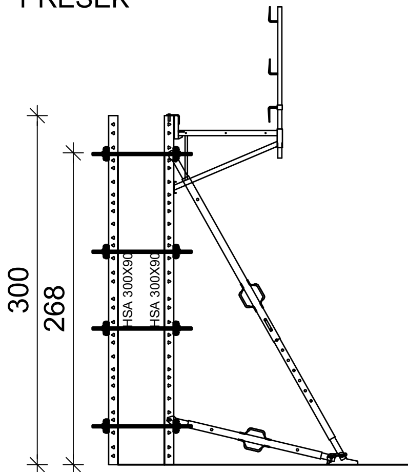
KARAKTERISTICAN PRESEK
