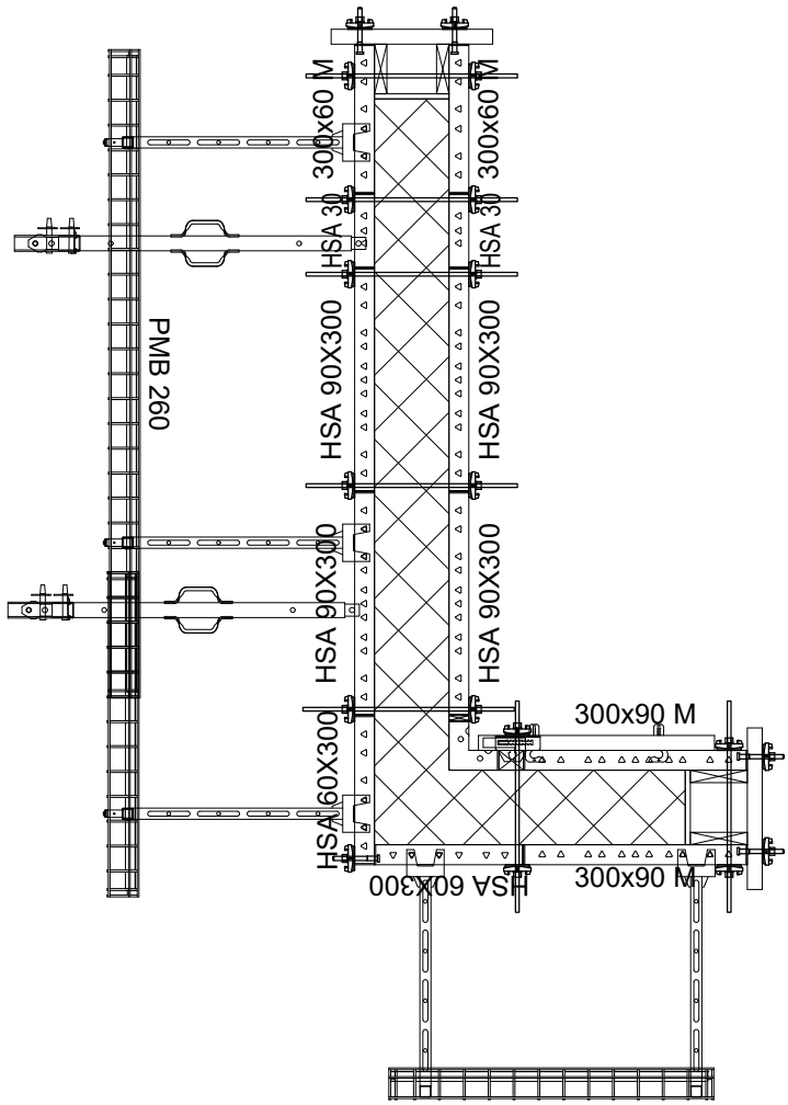
Oplata zidova 1:33
