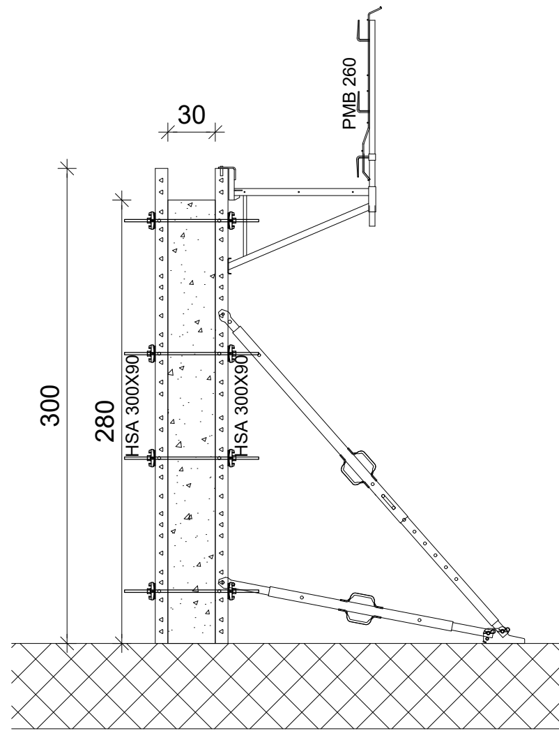
Presek 1-1 1:33
