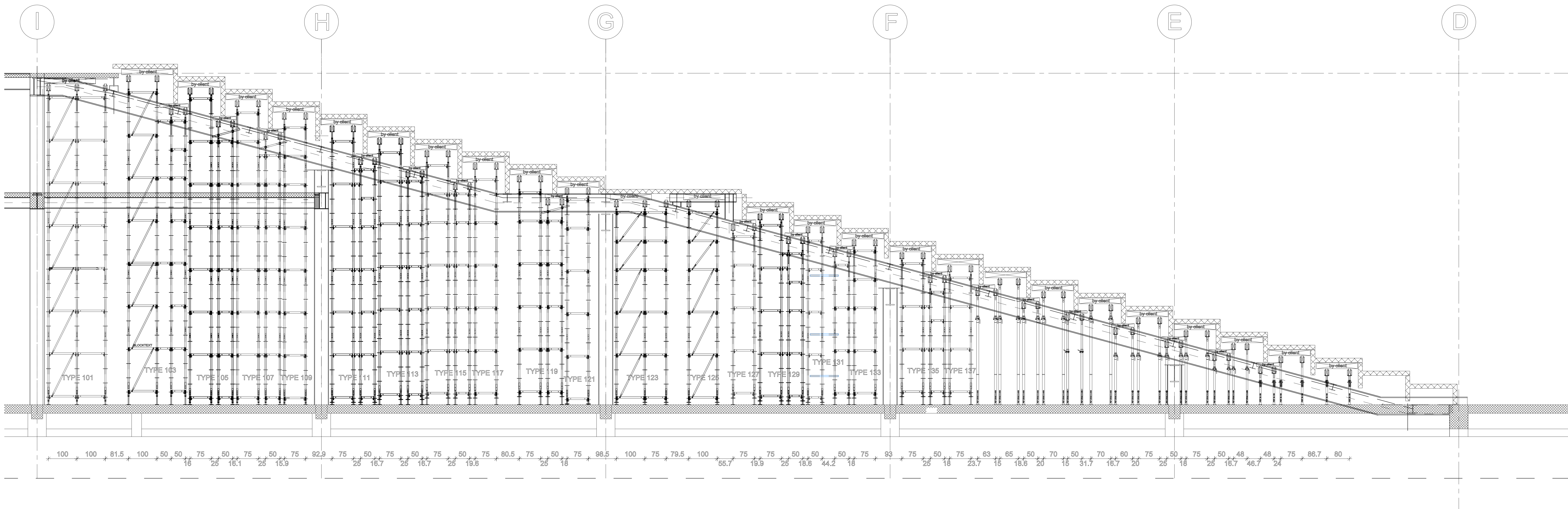
Longitudinal section 1:50
