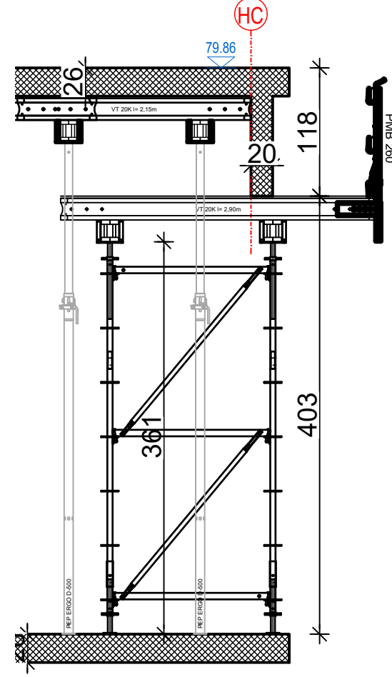
PRESEK B-B
